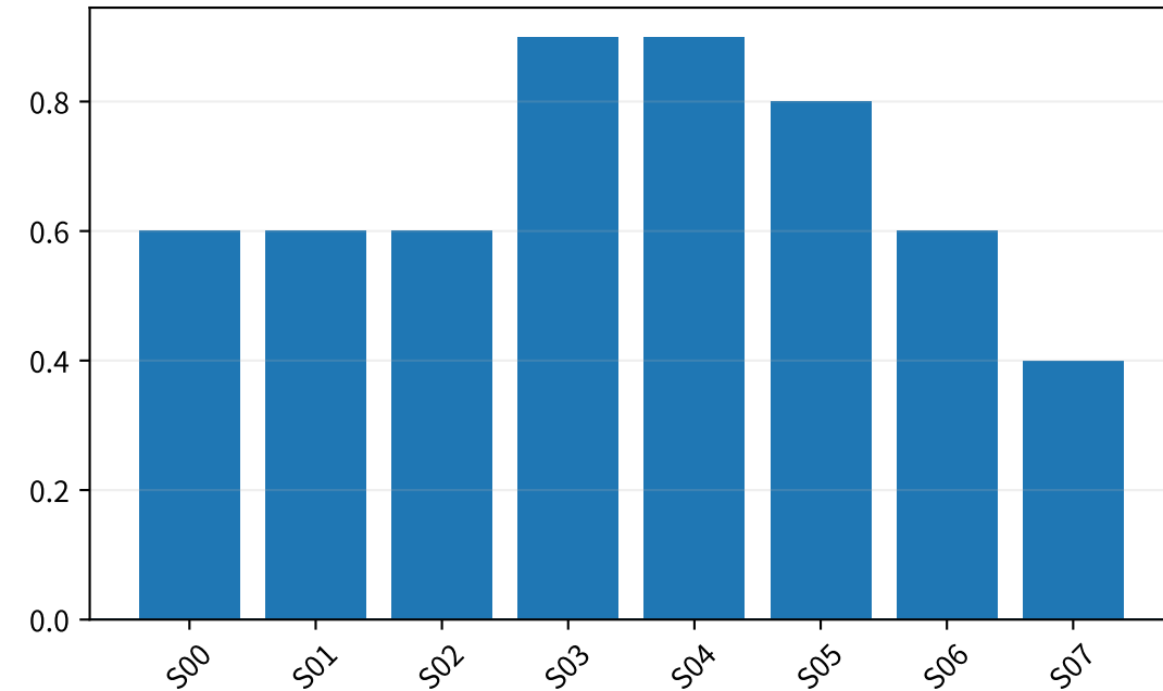
5分位単調性
