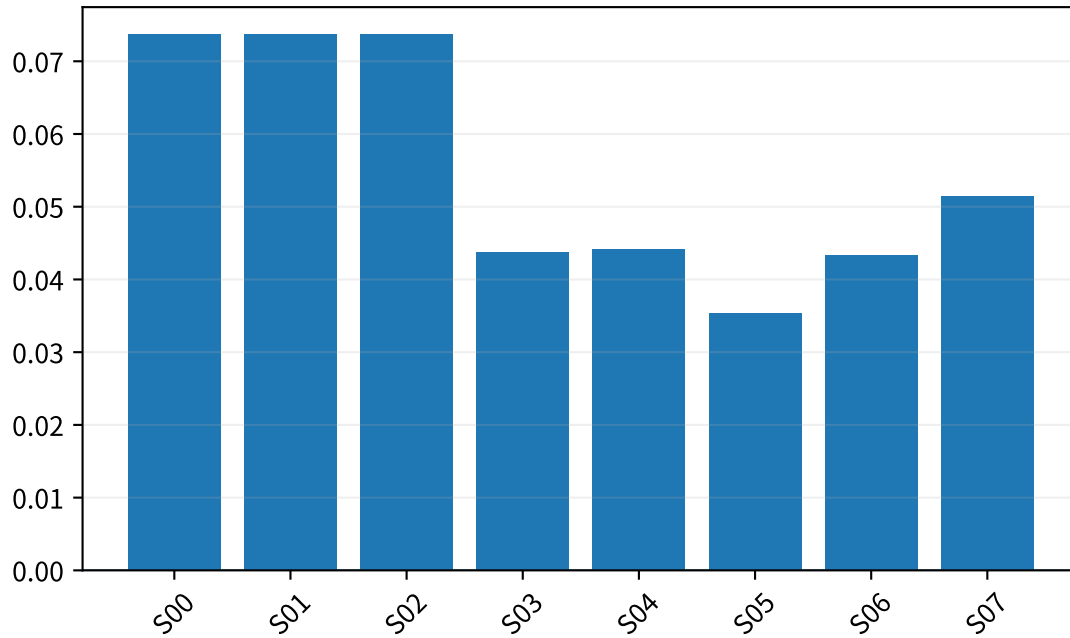
5分位単調性
